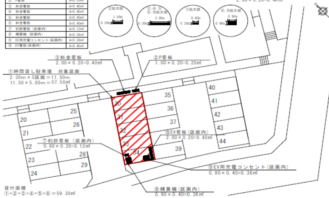
詳細図
