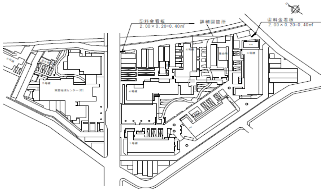
詳細図
