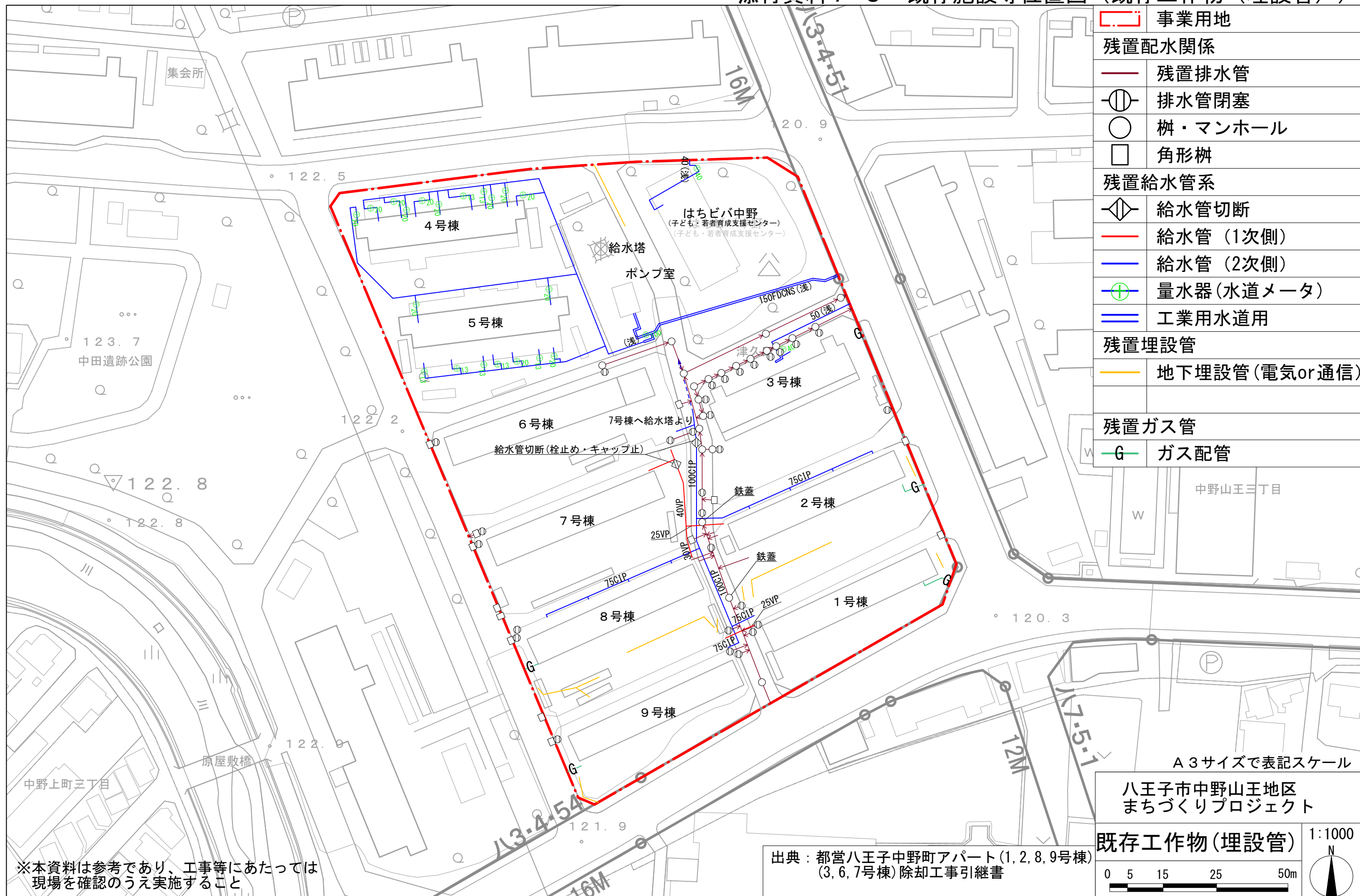
添付資料 7-3 既存施設等位置図（既存工作物（埋設管））
