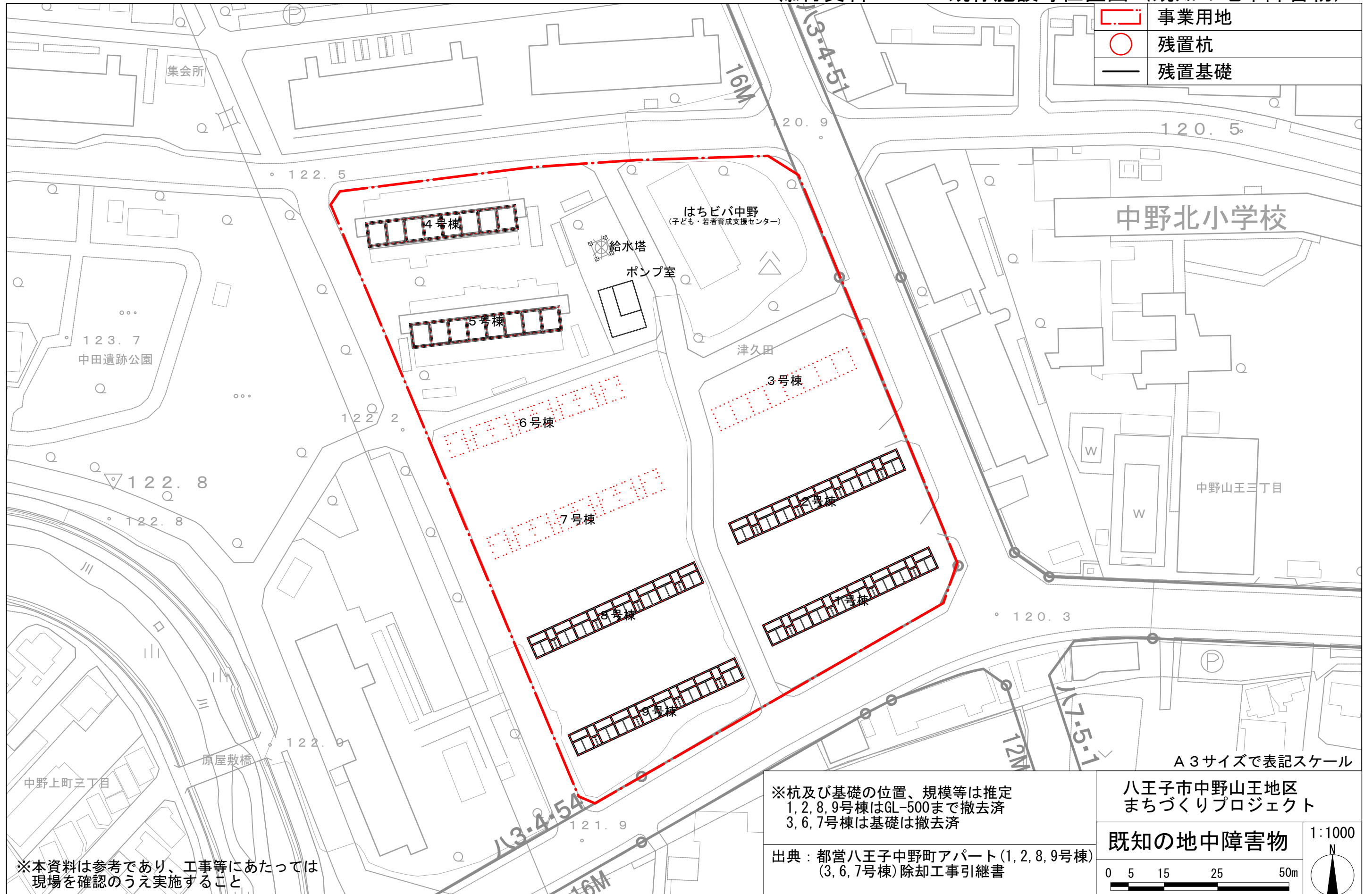
添付資料 7-2 既存施設等位置図（既知の地中障害物）
