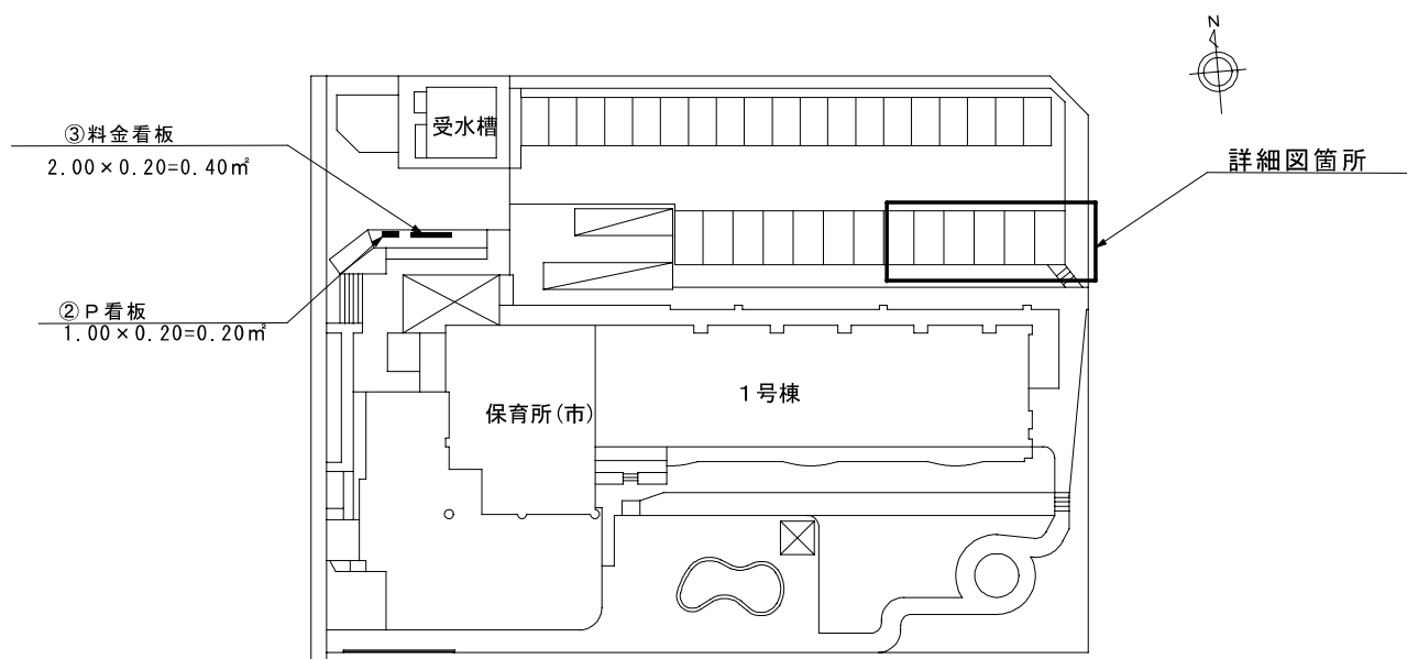
詳細図
