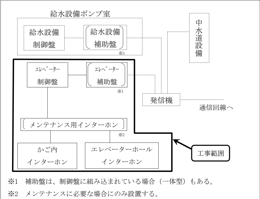
図 9.9.1 遠隔監視構成図
