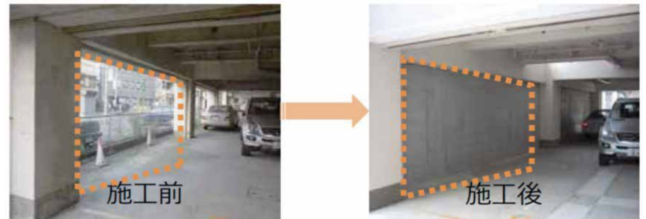
マンションの耐震改修の例 (耐震壁補強)
